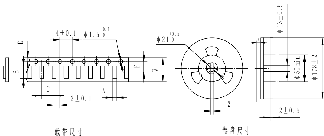
图3 编带尺寸
