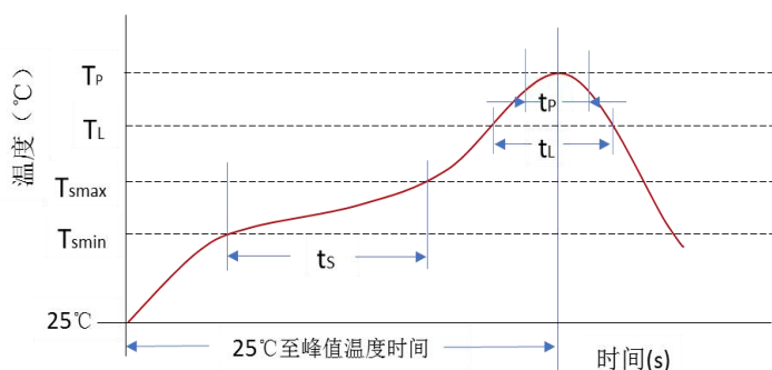
图 5 再流焊焊接曲线
