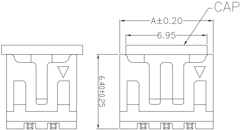
2P 视图
