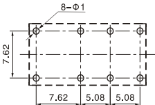
安装孔位图(底视图)
