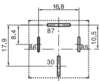
安装孔位图(底视图)
