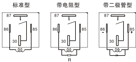
接线图(底视图)
