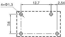
安装孔位图(底视图)
