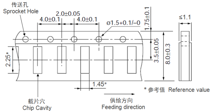
0805 系列 0805 series
