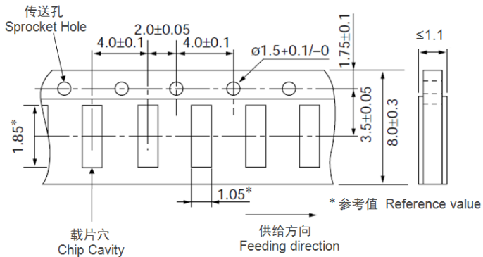
0603 系列 0603 series
