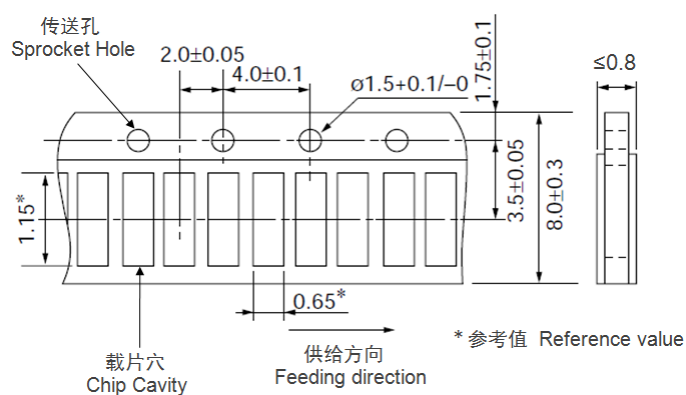
0805 系列 0805 series
