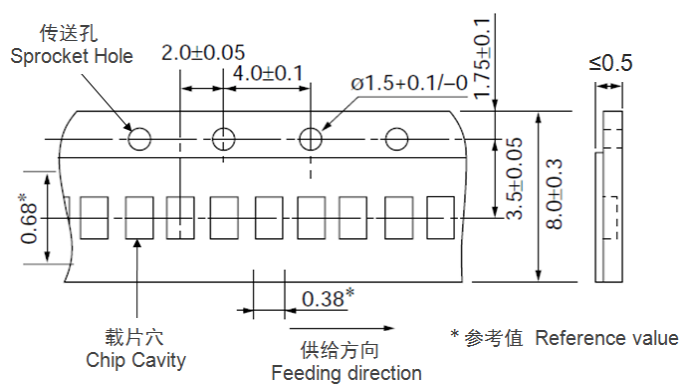
0603 系列 0603 series
