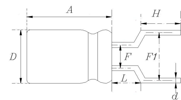
引线切脚成型 G 图
