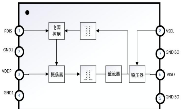
图 1 B0505ST8-W3原理框图
