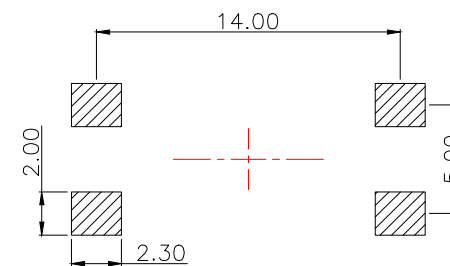
PCB.焊接图
