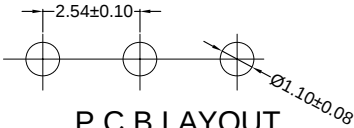
P.C.B LAYOUT
