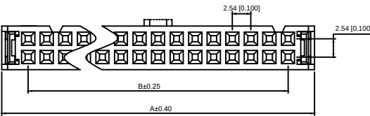
14P-64P 双槽
