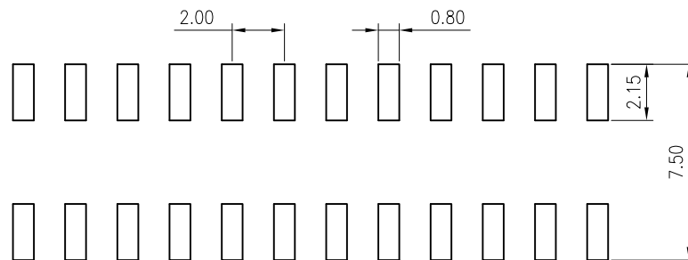
P.C.B. LAYOUT
