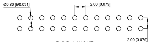
P.C.B LAYOUT
