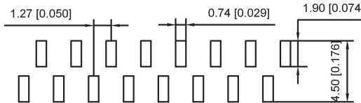
P.C.B LAYOUT(R2)
