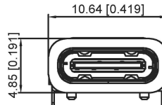
加防水圈示意图
