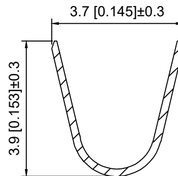
SEC:B-B
