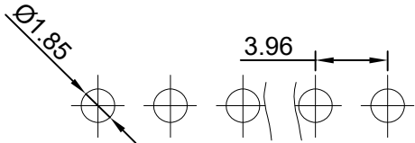
P.C.B Hole Layout
