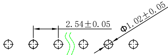
P.C.B Hole Layout
