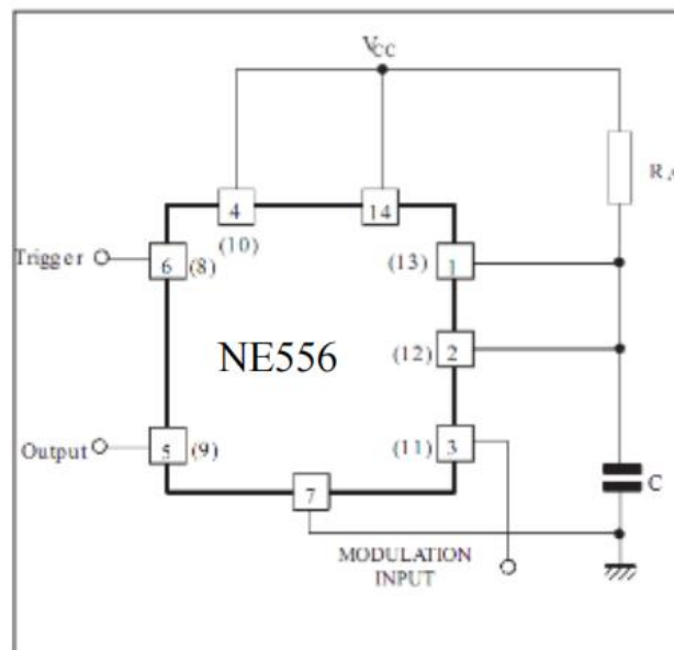
脉宽调制器
