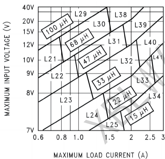
LM2596-5.0
