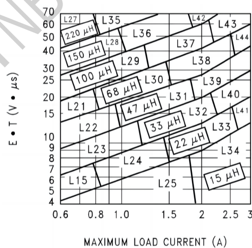
LM2596-ADJ
