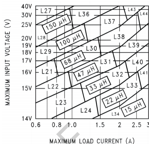
LM2596-12
