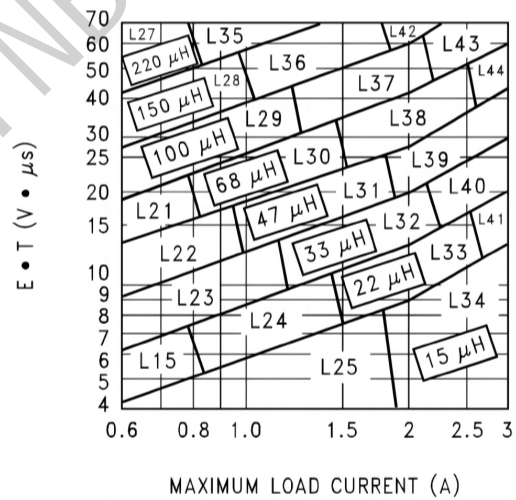
LM2596-ADJ
