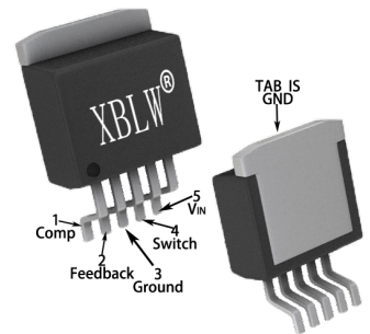
TO-263-5
