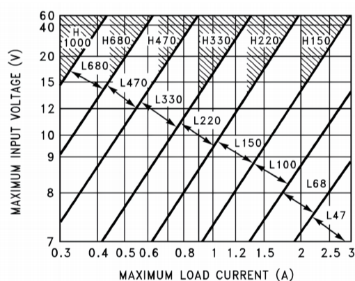
LM2576-5.0
