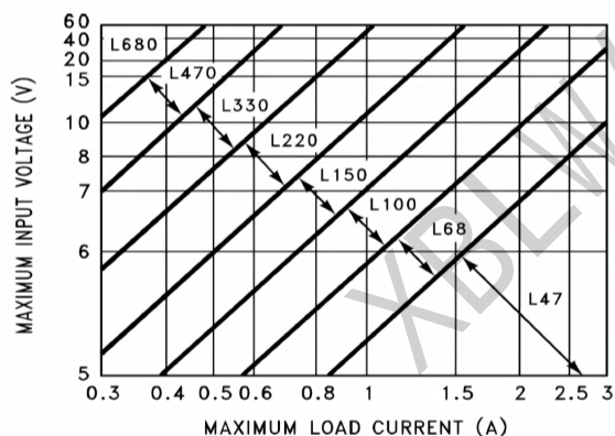
LM2576-3.3
