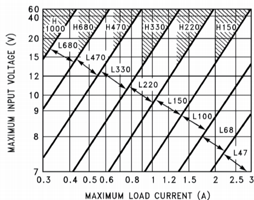
LM2576-5.0
