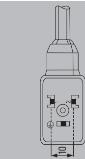
Contact gap 10 mm to DIN 43650 (ISO 6952) Type: VSBD
