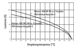
HDC-MHP100-Module im IP65-Gehäuse, Leiter H07V-K35:
