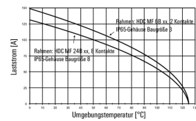
HDC-MHP100-Module im IP65-Gehäuse, Leiter H07V-K35:
