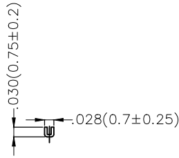
Section D-D
