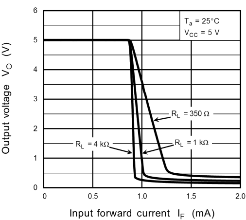
Fig. 12.2.8 V_O - I_F
