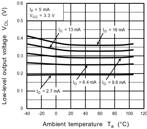
Fig. 12.2.5 V_{OL} - T_a
