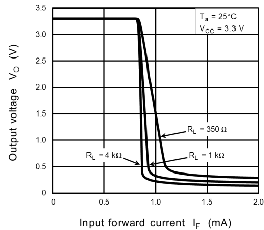
Fig. 12.2.7 V_O - I_F
