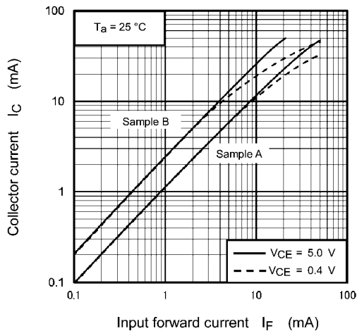
Fig. 11.9 I_C - I_F
