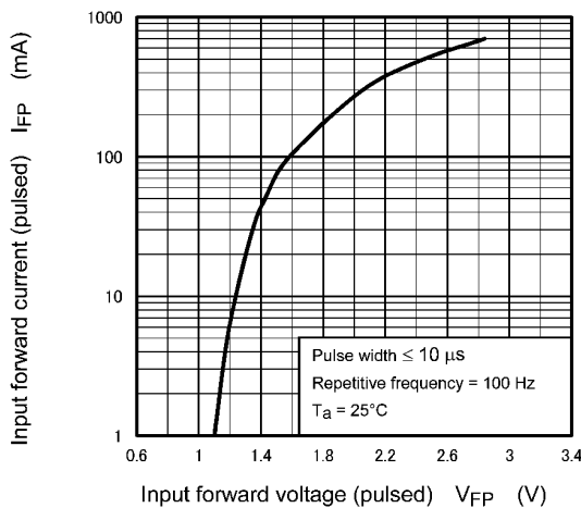
Fig. 11.6 I_{FP} - V_{FP}
