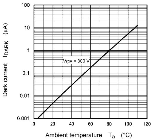
Fig. 11.11 I_{DARK} - T_a
