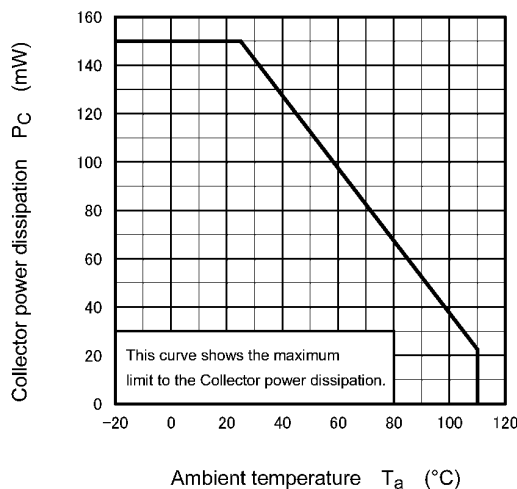
Fig. 11.2 P_C - T_a
