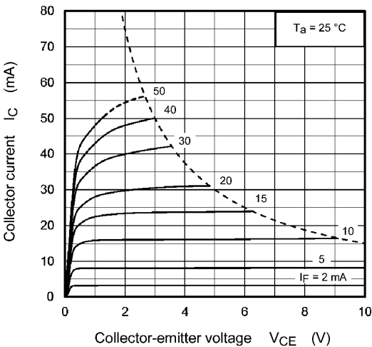
Fig. 11.7 I_C - V_{CE}
