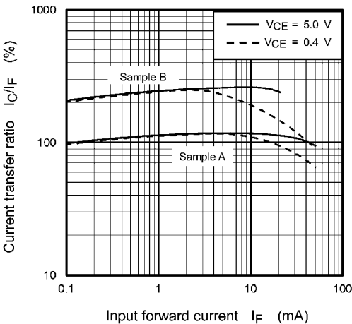
Fig. 11.10 I_C/I_F - I_F
