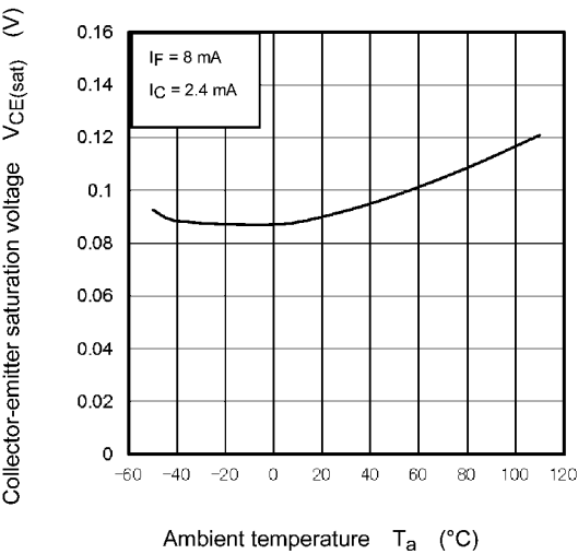
Fig. 11.12 V_{CE(sat)} - T_a
