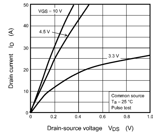
Fig. 7.1 I_D - V_{DS}
