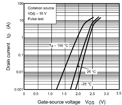
Fig. 7.2 I_D - V_{GS}
