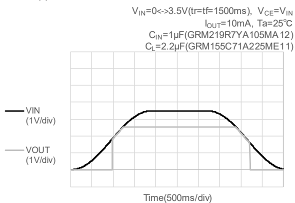
(16-1) V_{OUT(T)}=2.5V
