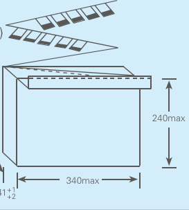
图3 盒装尺寸(mm)
