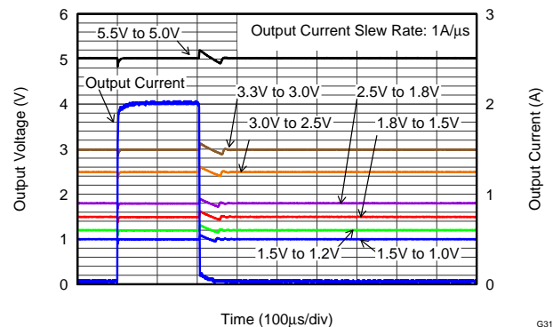
负载瞬态响应 (7 种不同输出)
