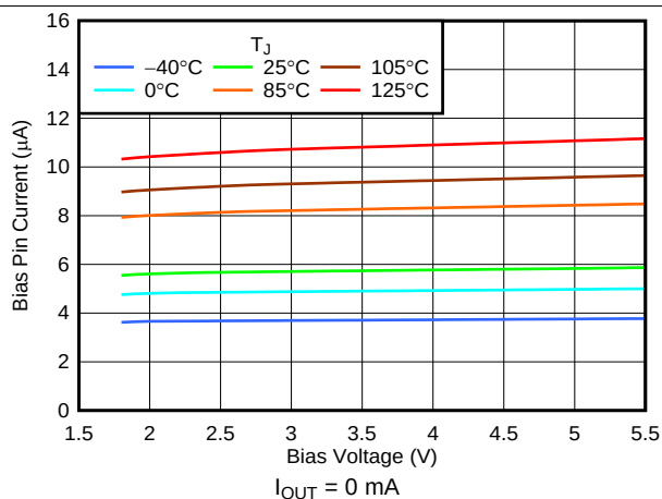
图 8. I_{Q(BIAS)} vs V_{BIAS} and Temperature
