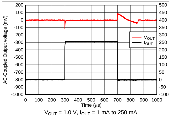
图 21. I_{OUT} Transient
