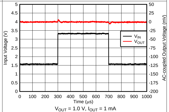
图 18. V_{IN} Transient
