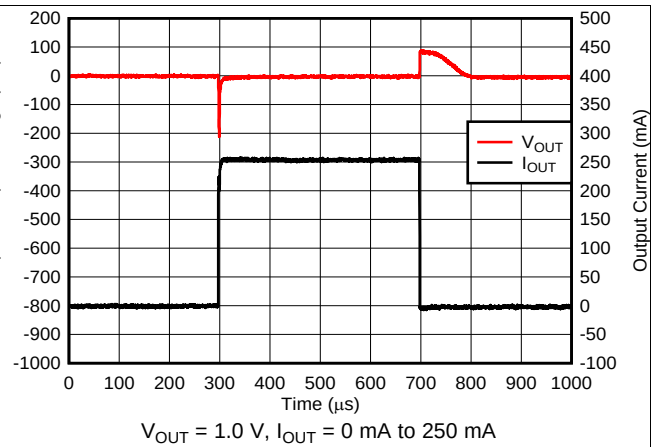
图 20. I_{OUT} Transient
