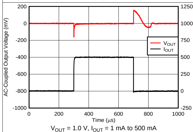
图 23. I_{OUT} Transient
