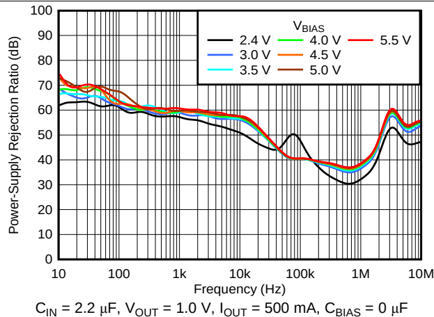
图 27. V_{BIAS} PSRR vs Frequency and V_{BIAS}
