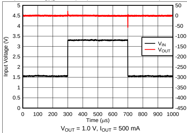
图 19. V_{IN} Transient
