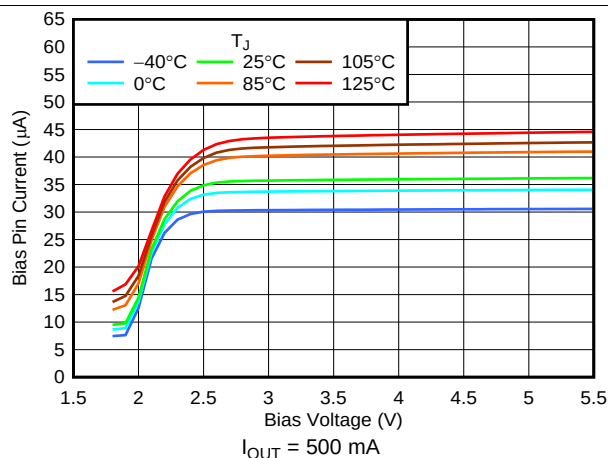
图 9. I_{Q(BIAS)} vs V_{BIAS} and Temperature
