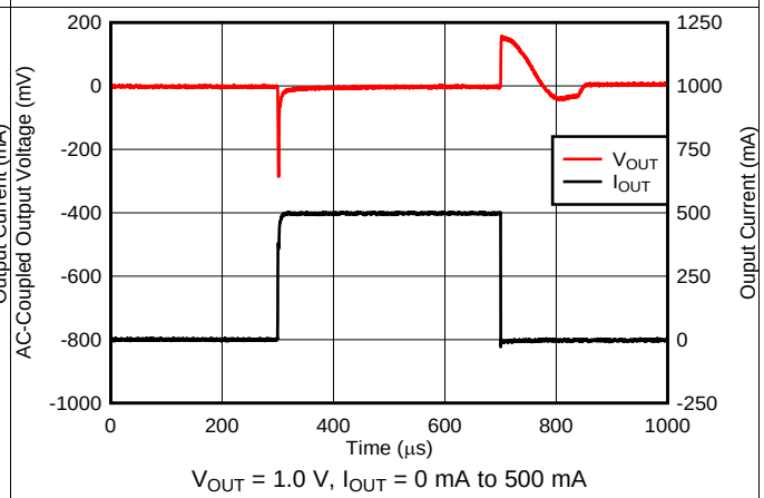
图 22. I_{OUT} Transient
