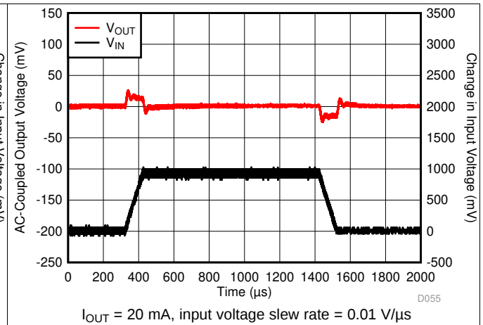
图 20. V_{IN} Transient
