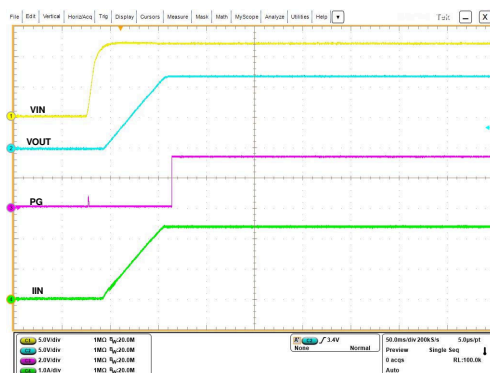
图 7-40. Input Hot-Plug
