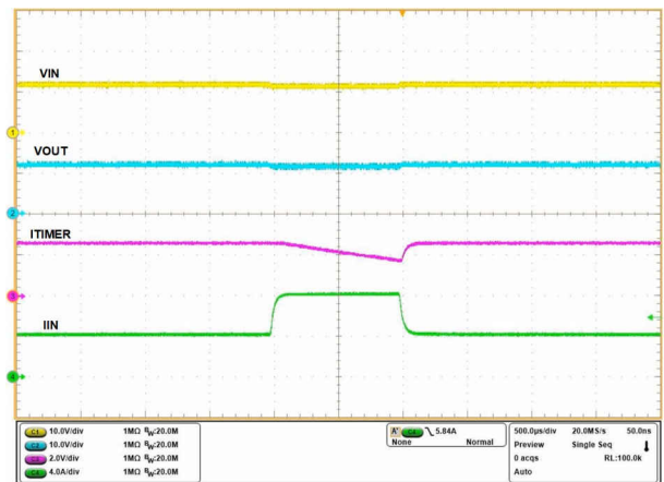
图 9-5. Transient Overload
