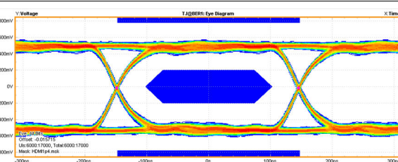
图 8-3. 3.4-Gbps HDMI 1.4 TP1 Eye Diagram TPD1E05U06
