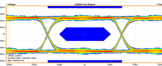
图 8-5. 3.4-Gbps HDMI 1.4 TP1 Eye Diagram TPD6E05U06
