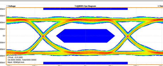
图 8-7. 6-Gbps HDMI 2.0 (TP1) Eye Diagram TPD1E05U06
