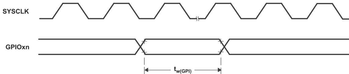
图 7-10. 通用输入时序
