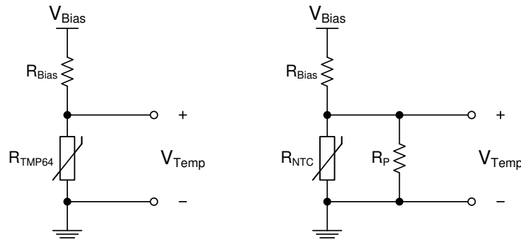
图 9-4. TMP64-Q1 与带线性化电阻 ( R_P ) 分压器电路的 NTC 间的关系
