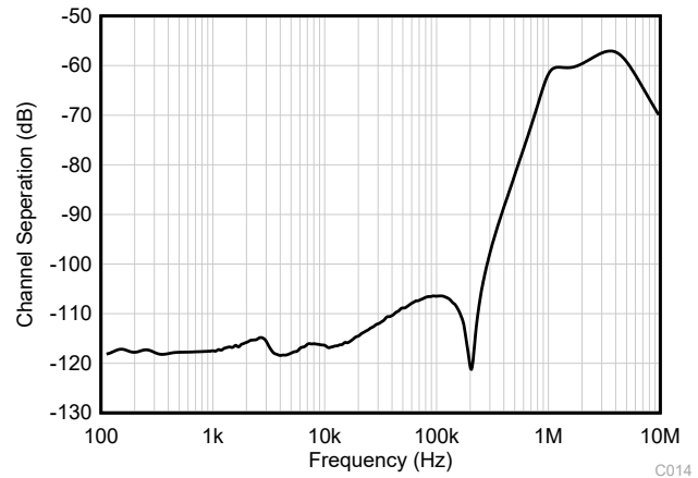
图 6-40. 通道隔离与频率间的关系
