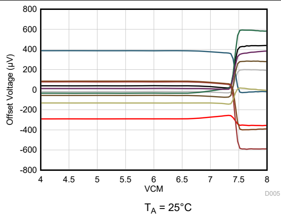
图 6-6. 失调电压与共模电压间的关系 (切换区域)
