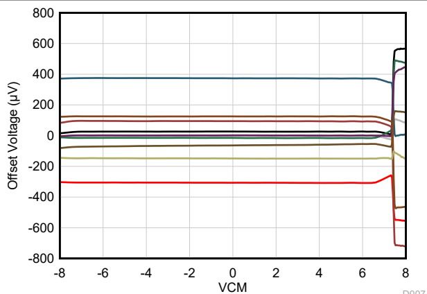
图 6-8. 失调电压与共模电压间的关系
