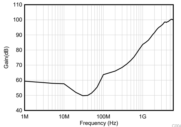
图 6-41. EMIRR (电磁干扰抑制比) 输入与频率间的关系
