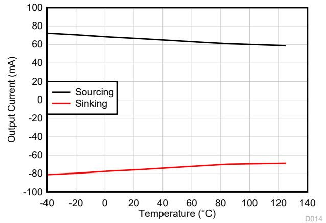
图 6-38. 短路电流与温度间的关系
