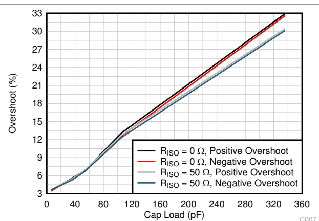
图 7-4. 小信号过冲与容性负载之间的关系 (10mV 输出阶跃, G = -1 )
