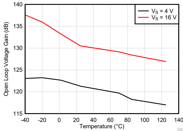
图 6-25. 开环电压增益与温度间的关系 (dB)
