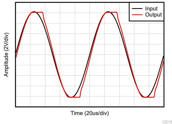
图 7-7. 无相位反转
