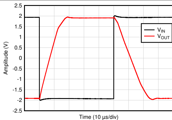
图 7-38. 大信号阶跃响应
