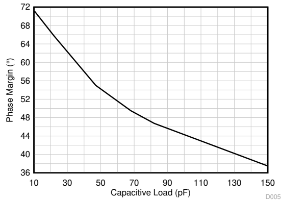
图 7-31. 相位裕度与容性负载间的关系
