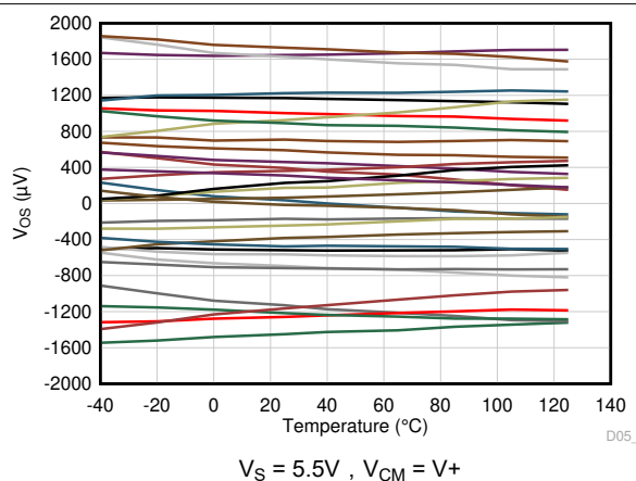
图 7-4. 输入失调电压与温度间的关系
