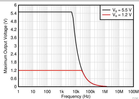
图 7-39. 最大输出电压与频率间的关系
