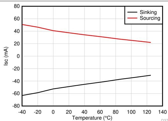
图 7-40. 短路电流与温度间的关系
