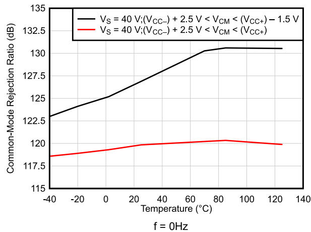
图 6-15. CMRR 与温度间的关系 (dB)
