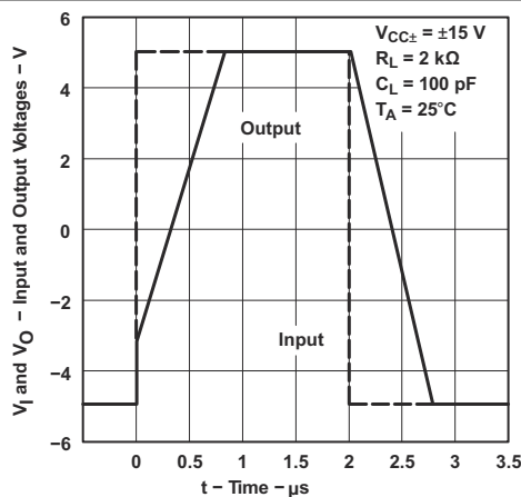
图 6-57. 电压跟随器大信号脉冲响应
