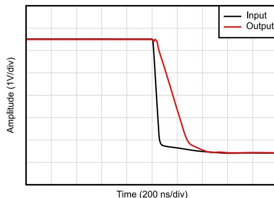
图 6-32. 小信号阶跃响应, 下降
