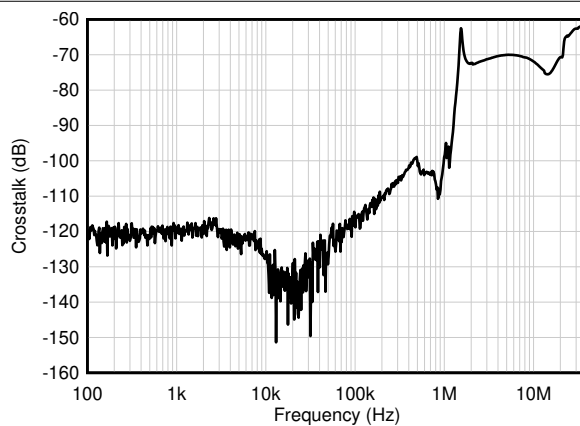
图 6-42. 通道隔离与频率间的关系
