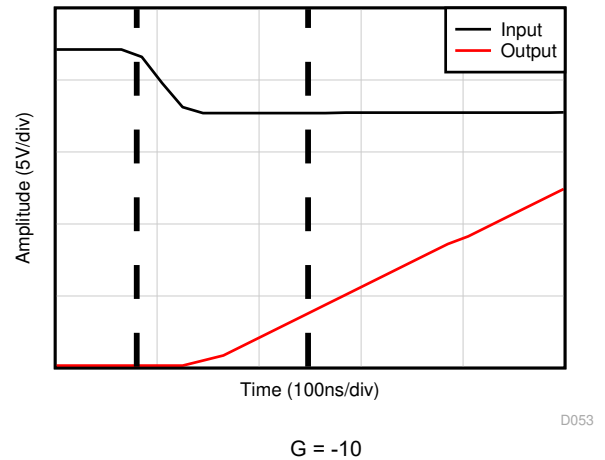
图 6-36. 负过载恢复
