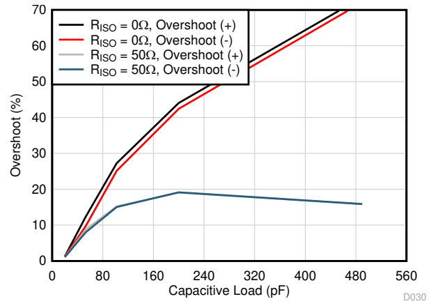
图 6-32. 小信号过冲与容性负载间的关系
