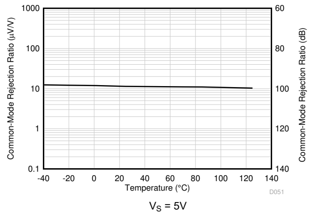
图 6-22. CMRR 与温度间的关系
