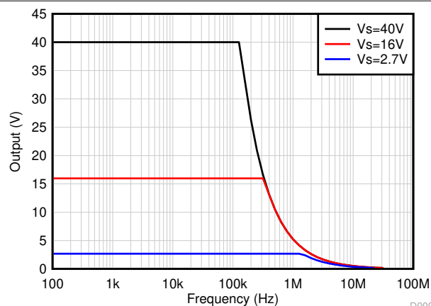
图 6-41. 最大输出电压与频率间的关系
