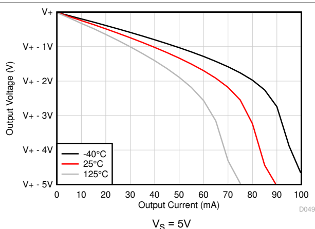
图 6-18. 输出电压摆幅与输出电流 (拉电流) 间的关系
