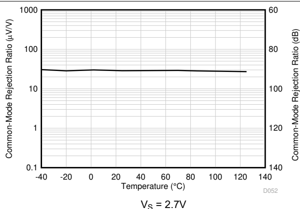
图 6-23. CMRR 与温度间的关系
