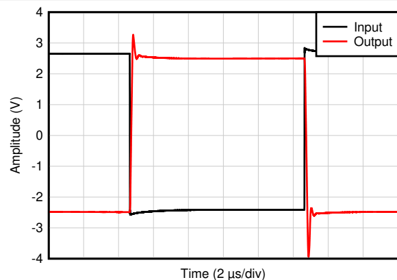
C_L = 20\text{pF} , G = -1 , 5\text{V}_{pp} 阶跃响应
