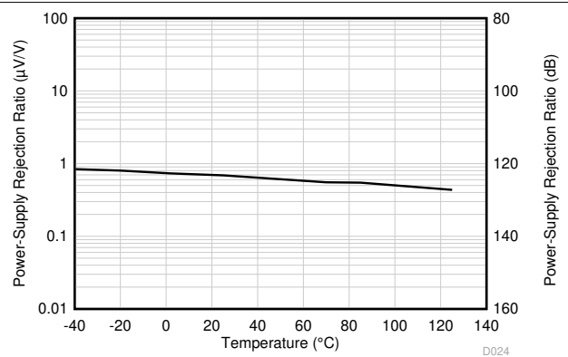
图 6-24. PSRR 与温度间的关系
