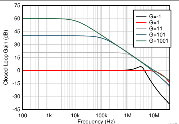
图 6-12. 闭环增益与频率间的关系
