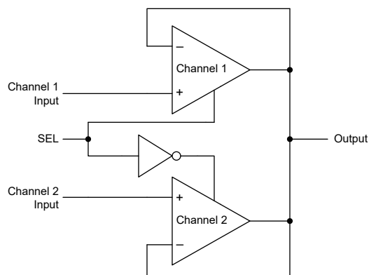
图 8-3. 高电压缓冲多路复用器
