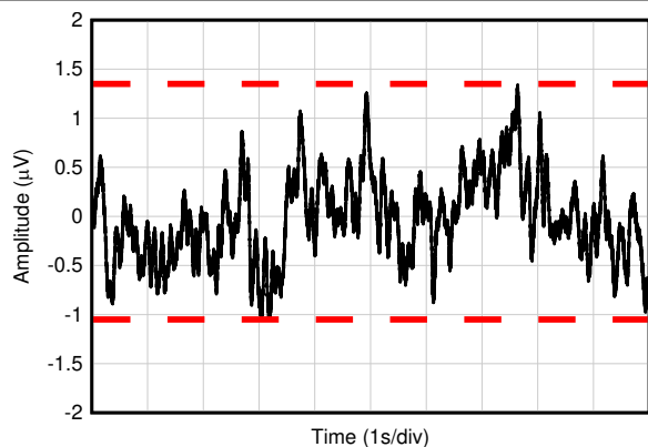
图 6-25. 0.1Hz 至 10Hz 噪声
