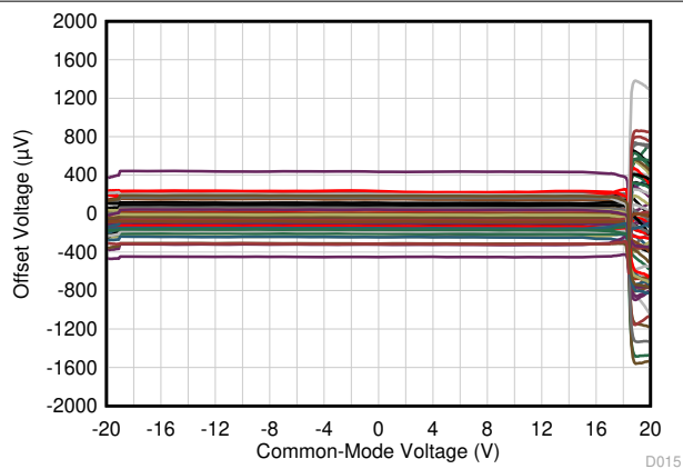
T_A = 25^\circ\text{C} 来自 74 个放大器的数据
