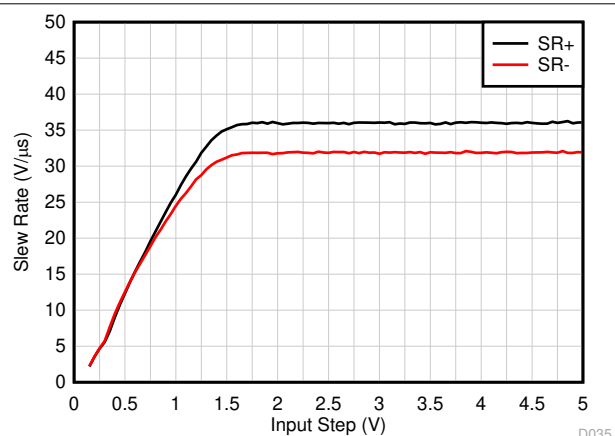
图 6-15. 压摆率与输入阶跃电压间的关系
