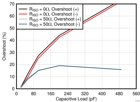
图 7-5. 小信号过冲与容性负载之间的关系 ( 20\text{mV}_{\text{pp}} 输出阶跃, G = +1 )
