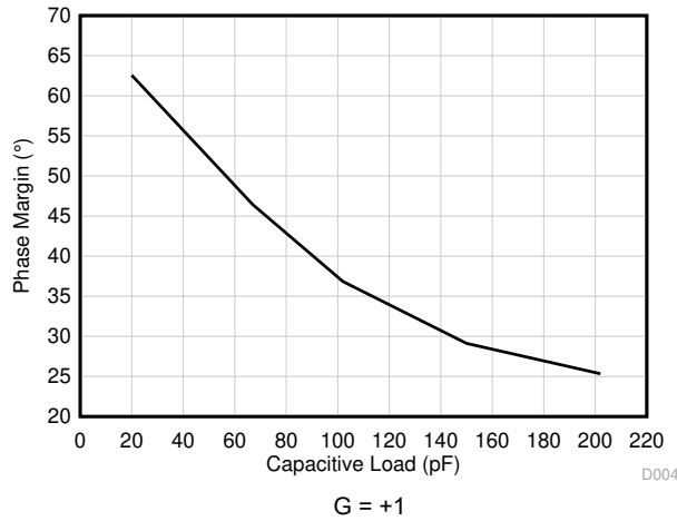
图 6-33. 相位裕度与容性负载间的关系
