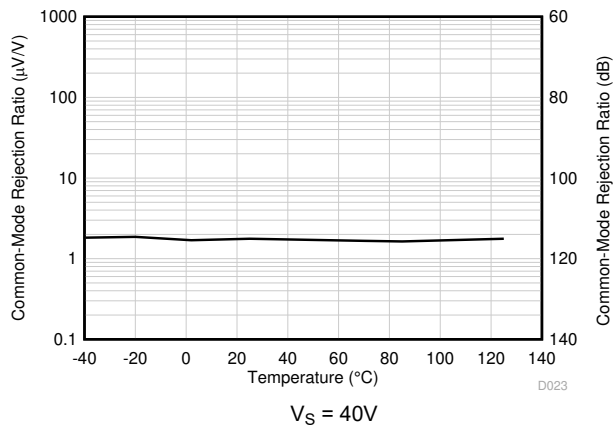
图 6-21. CMRR 与温度间的关系
