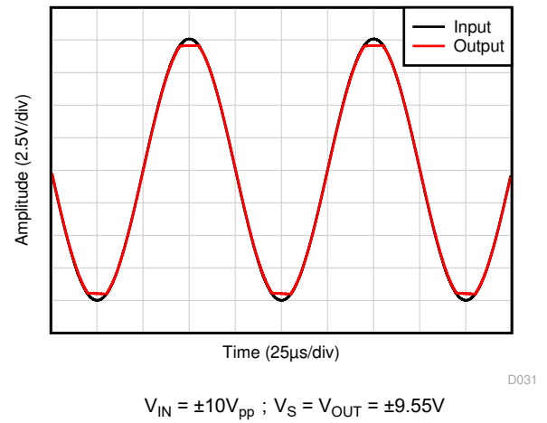
图 6-34. 无相位反转
