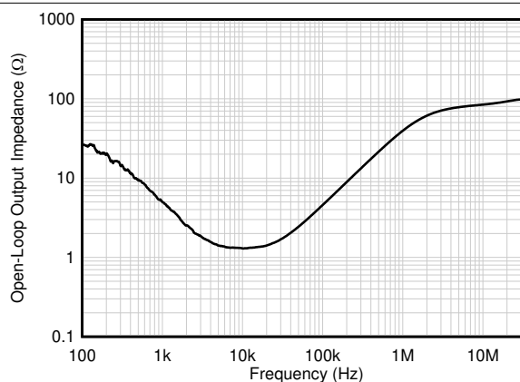
图 6-30. 开环输出阻抗与频率间的关系
