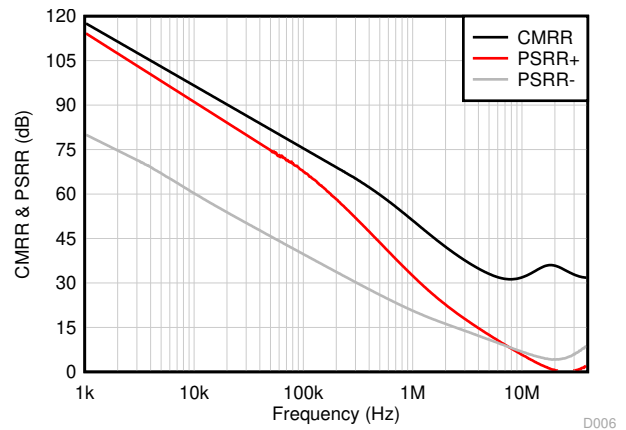
图 6-20. CMRR 和 PSRR 与频率间的关系
