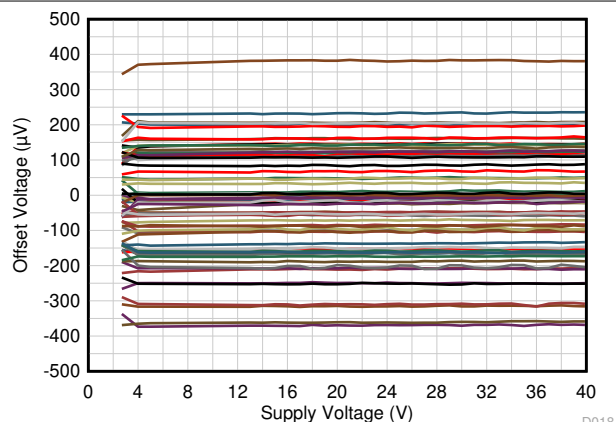
V_{CM} = V_S 来自 74 个放大器的数据
