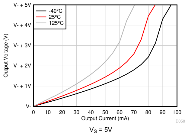
图 6-19. 输出电压摆幅与输出电流 ( 灌电流 ) 间的关系
