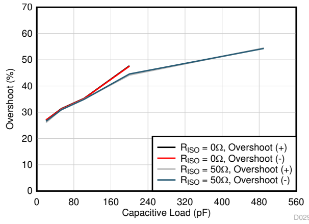
图 6-31. 小信号过冲与容性负载间的关系
