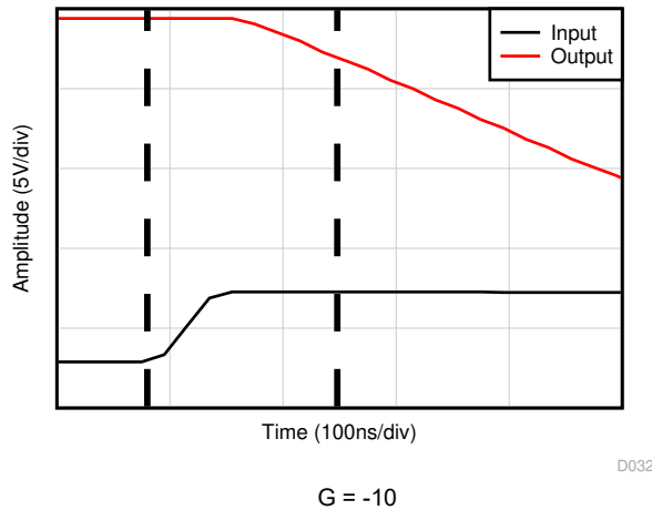
图 6-35. 正过载恢复
