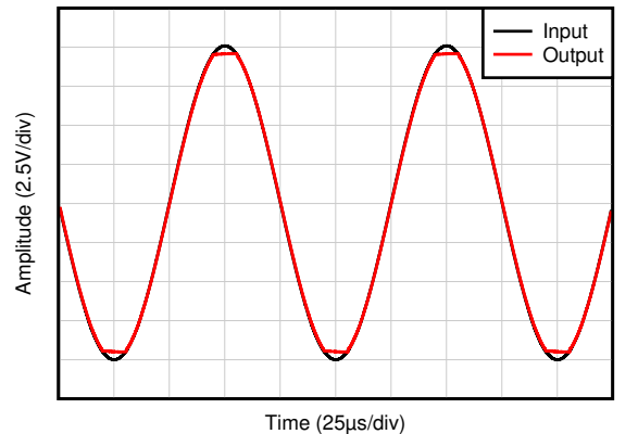
图 7-9. 无相位反转
