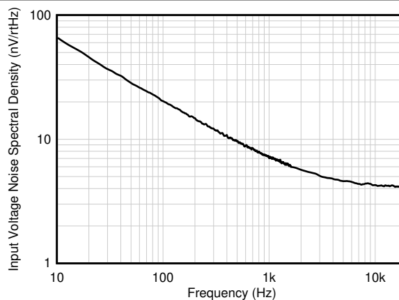
图 6-26. 输入电压噪声频谱密度与频率间的关系
