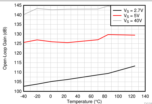
图 6-29. 开环电压增益与温度间的关系 (dB)
