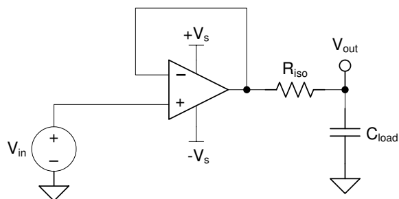
图 7-7. 使用 OPA992 扩展容性负载驱动
