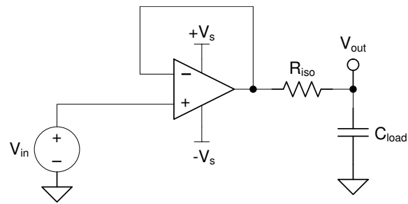
图 7-7. 使用 OPAx991-Q1 扩展容性负载驱动
