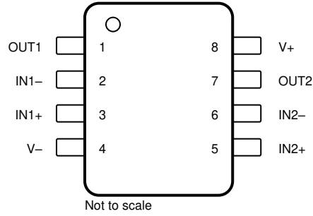
图 5-2. OPA2991-Q1 D 和 DGK 封装 8 引脚 SOIC 和 VSSOP 顶视图
