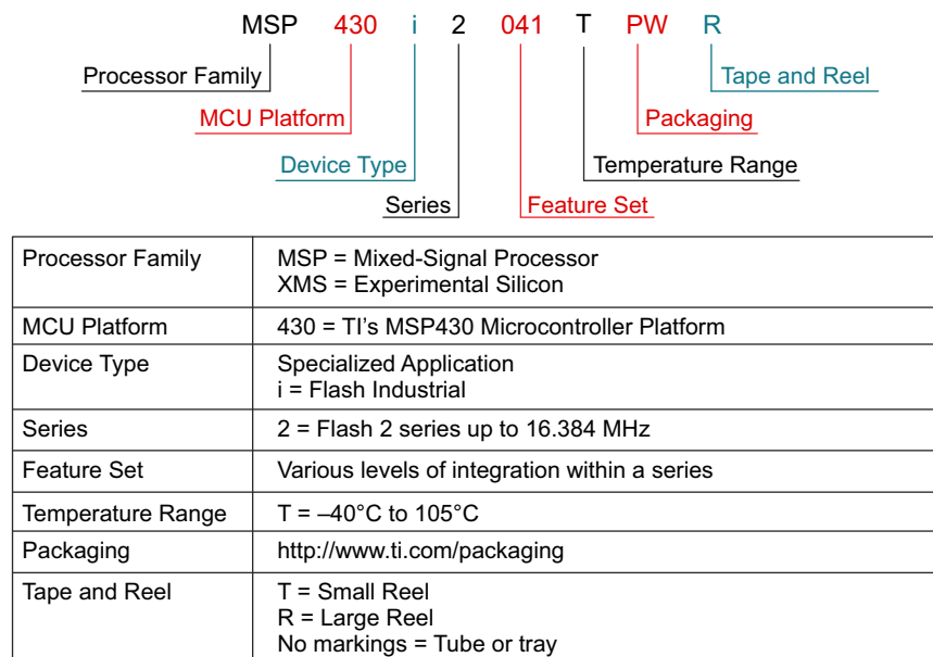
图 11-1. Device Nomenclature
