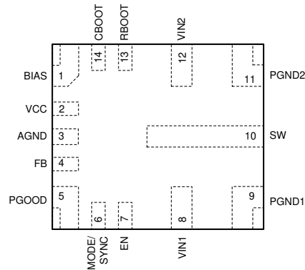
图 7-1. RJR Package 14-Pin VQFN-HR Top View
