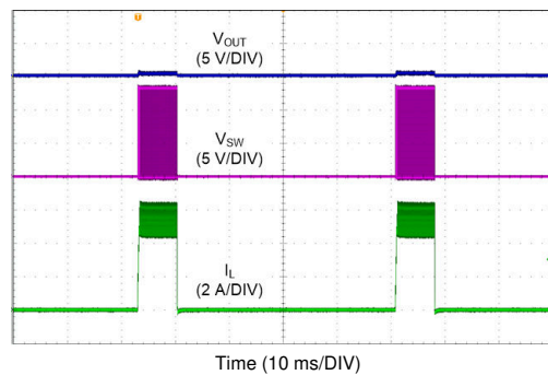
图 10-20. LM62440-Q1 Short Circuit Protection
