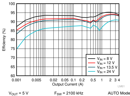
图 10-7. LM62440-Q1 Efficiency
