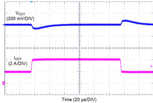
图 10-24. LM62440-Q1 Load Transient
