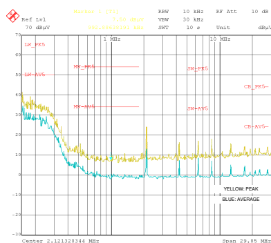
传导 EMI: V_{\text{OUT}}=5\text{V} , f_{\text{SW}}=2100\text{kHz}
