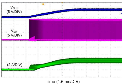
图 10-19. LM62440-Q1 Start-up with 3.25-A
