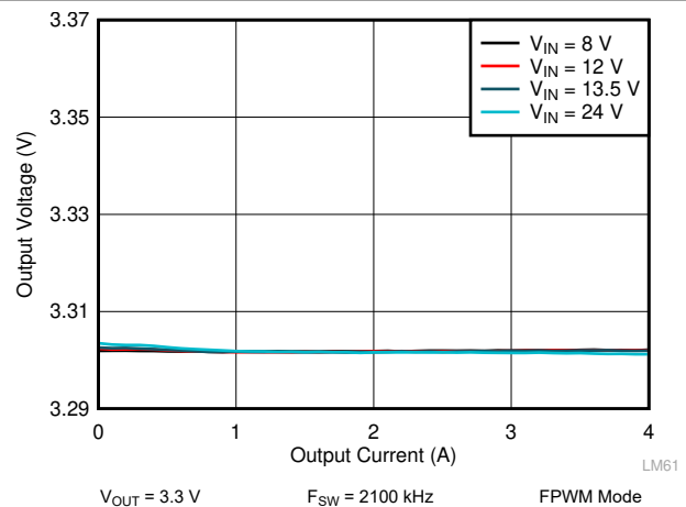
图 10-10. LM62440-Q1 Load and Line Regulation
