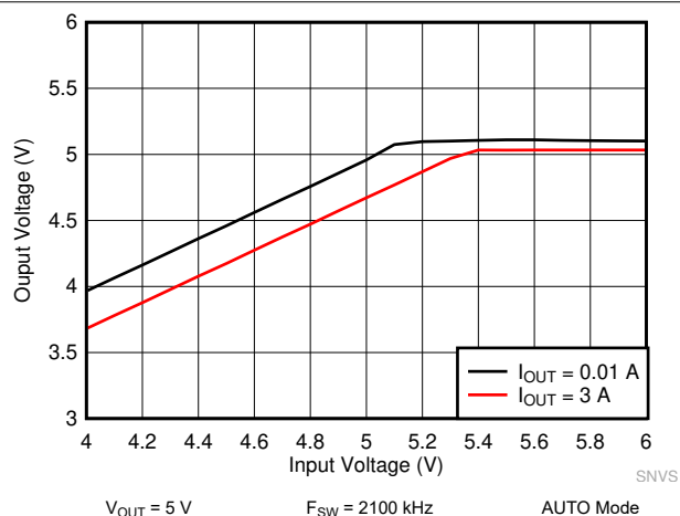
图 10-14. LM62440-Q1 Dropout Curve
