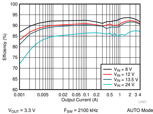
图 10-5. LM62440-Q1 Efficiency
