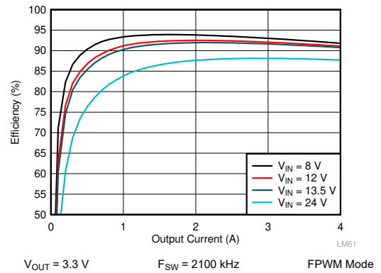
图 10-6. LM62440-Q1 Efficiency
