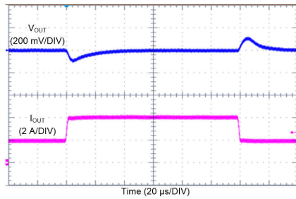
图 10-23. LM62440-Q1 Load Transient
