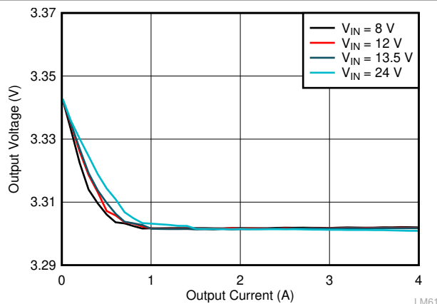
图 10-9. LM62440-Q1 Load and Line Regulation
