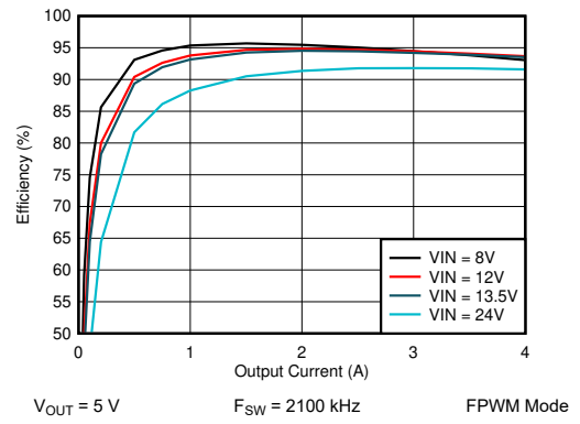
图 10-8. LM62440-Q1 Efficiency
