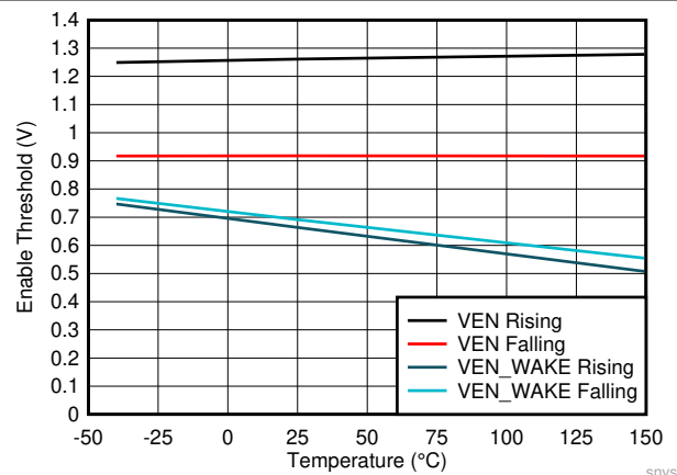
图 8-7. Enable Thresholds
