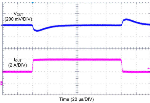
图 10-25. LM62440-Q1 Load Transient
