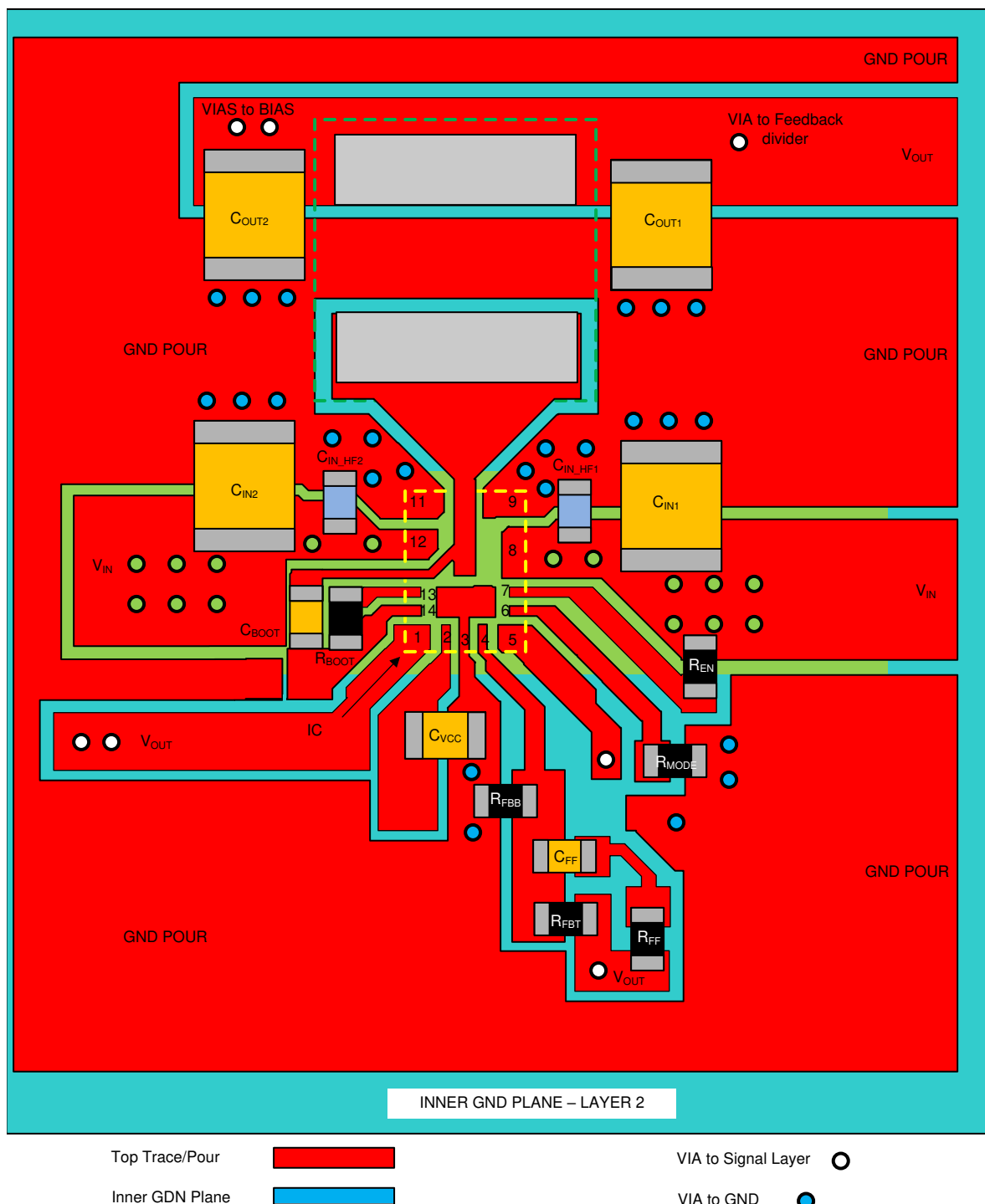
图 12-2. Layout Example
