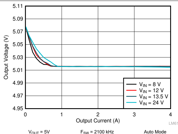
图 10-11. LM62440-Q1 Load and Line Regulation
