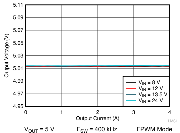
图 10-14. LM61440-Q1 Load and Line Regulation
