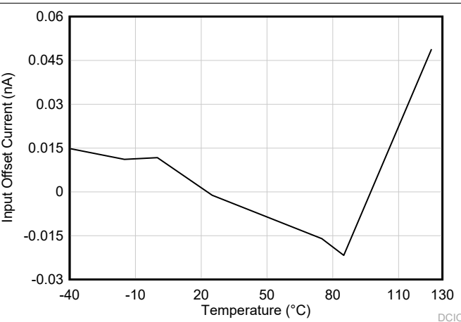
图 6-10. 输入失调电流与温度间的关系
