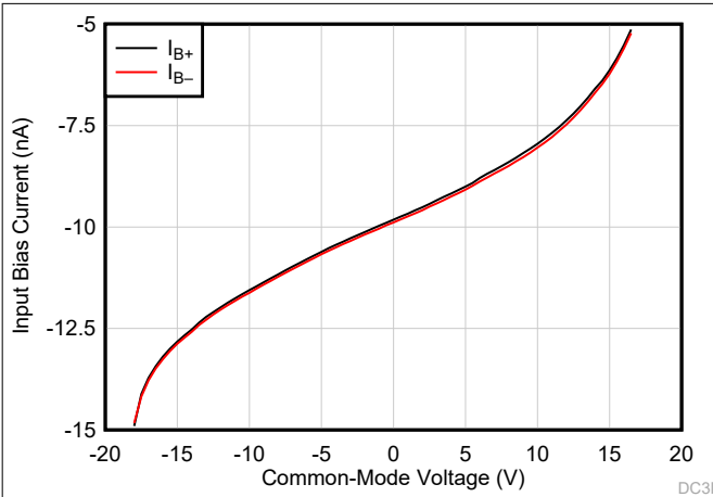
图 6-7. 输入偏置电流与共模电压间的关系
