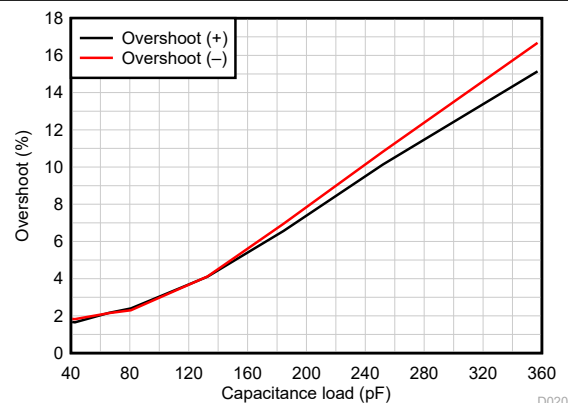
图 6-26. 小信号过冲与容性负载间的关系
