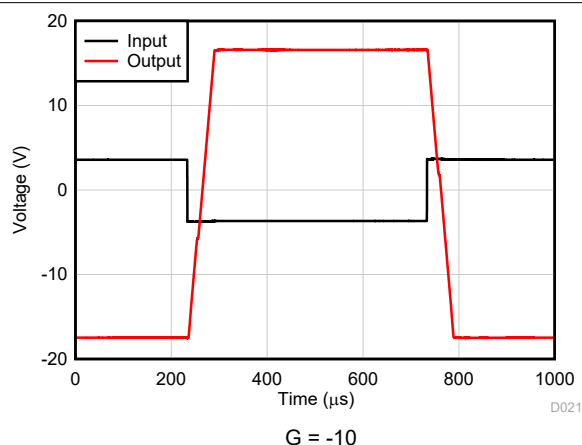
图 6-28. 过载恢复
